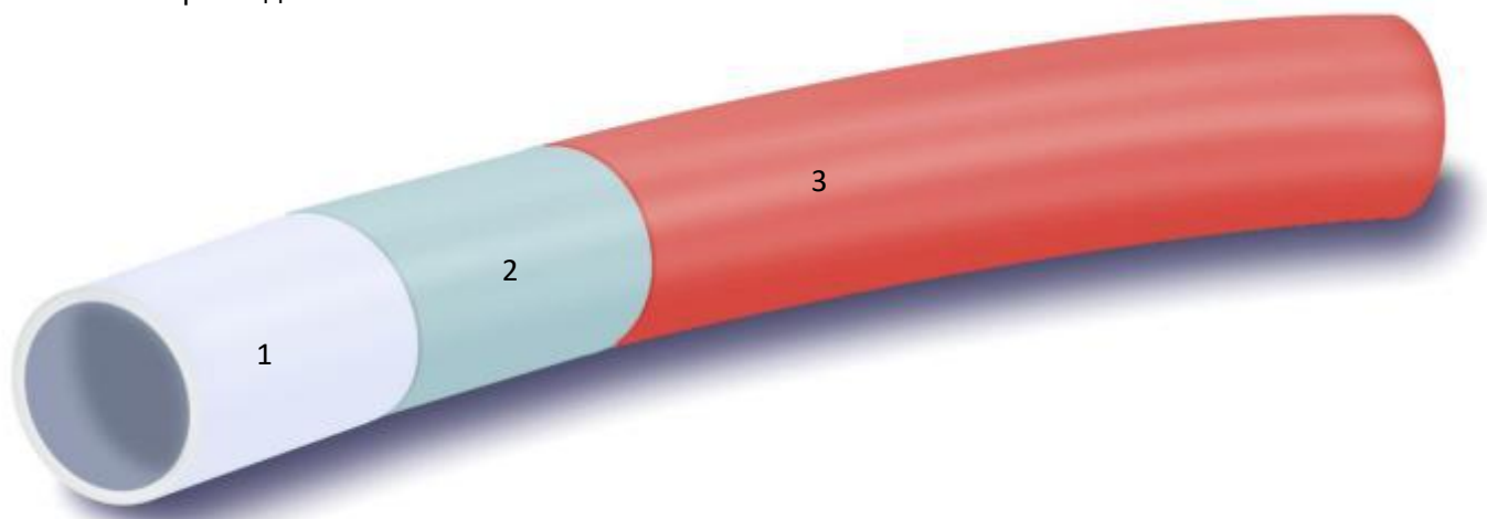
Рисунок 1 – Общий вид трубы РЕ-Ха EVOH RITABLE (теплый пол).
