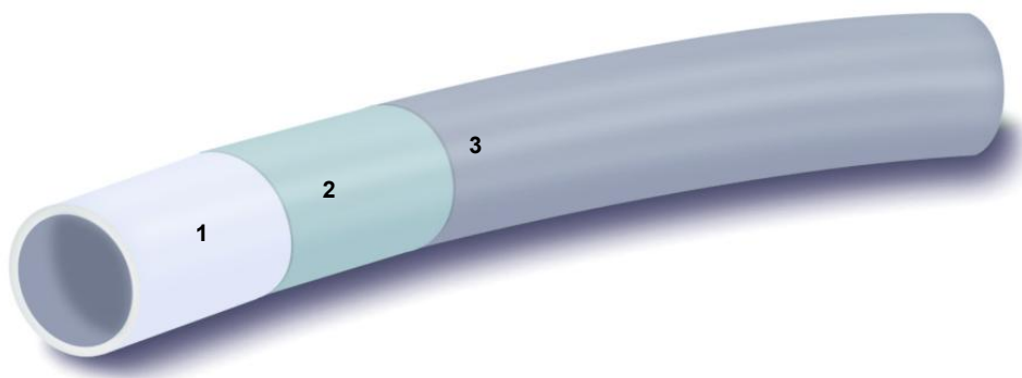
Рисунок 1 – Общий вид трубы PE-Ха EVOH RITABLE 1 .
